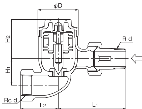
TS-1S &lt;Straight type&gt;
