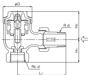
TS-1A &lt;Angle type&gt;
